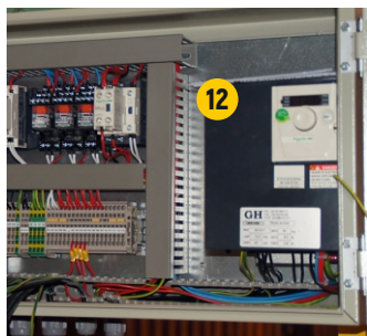
9 / Armário elétrico da ponte
